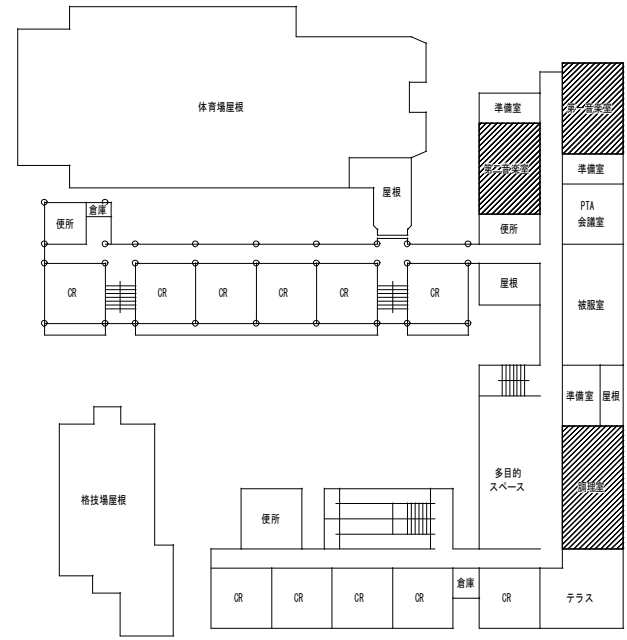
3階平面図 1/500
