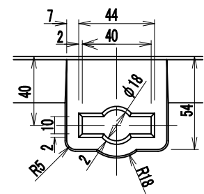
C部詳細図
