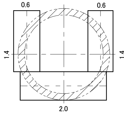
内径 1800mm
