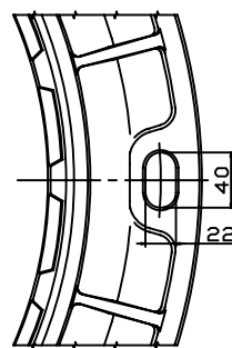
アンカー穴詳細
