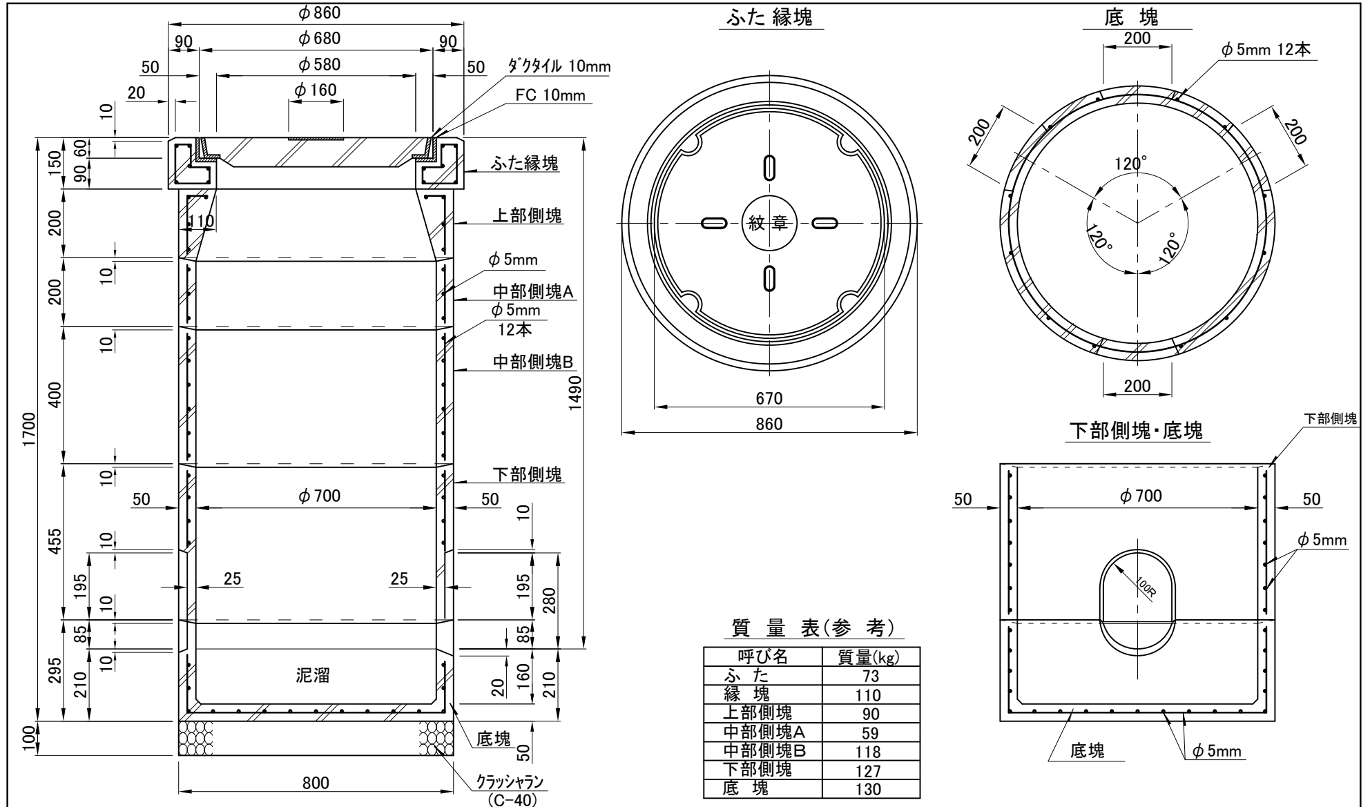
タイプ9接続雨水枈構造図 (φ700)
