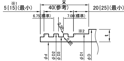
継手差し口部詳細図 (Coupling Inlet Detail)
