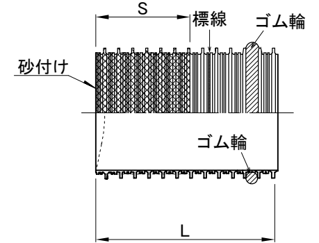
下流用マンホール継手 (略号MSA-PRP)
