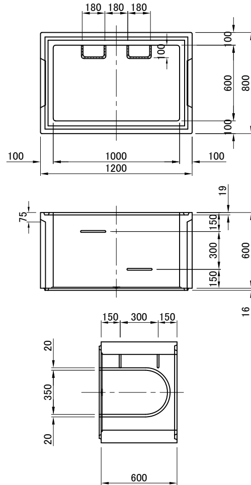
Eブロック構造図 H=600
