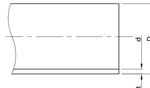
副管用90度支管直管部共通寸法
