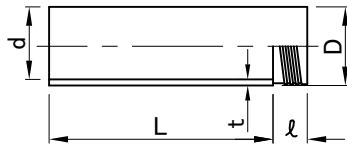
先頭管 (Front Pipe)
