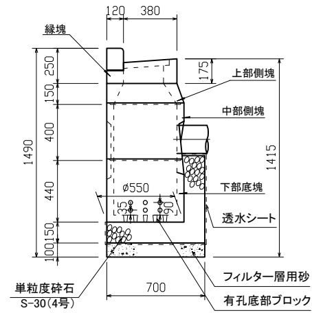
B-B 断面図
