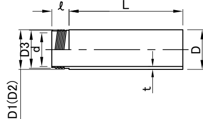
最終管 (Final Pipe)
