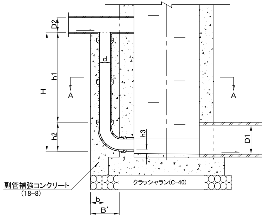
断面図(1)
