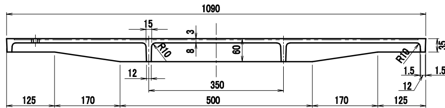
A-A断面図
