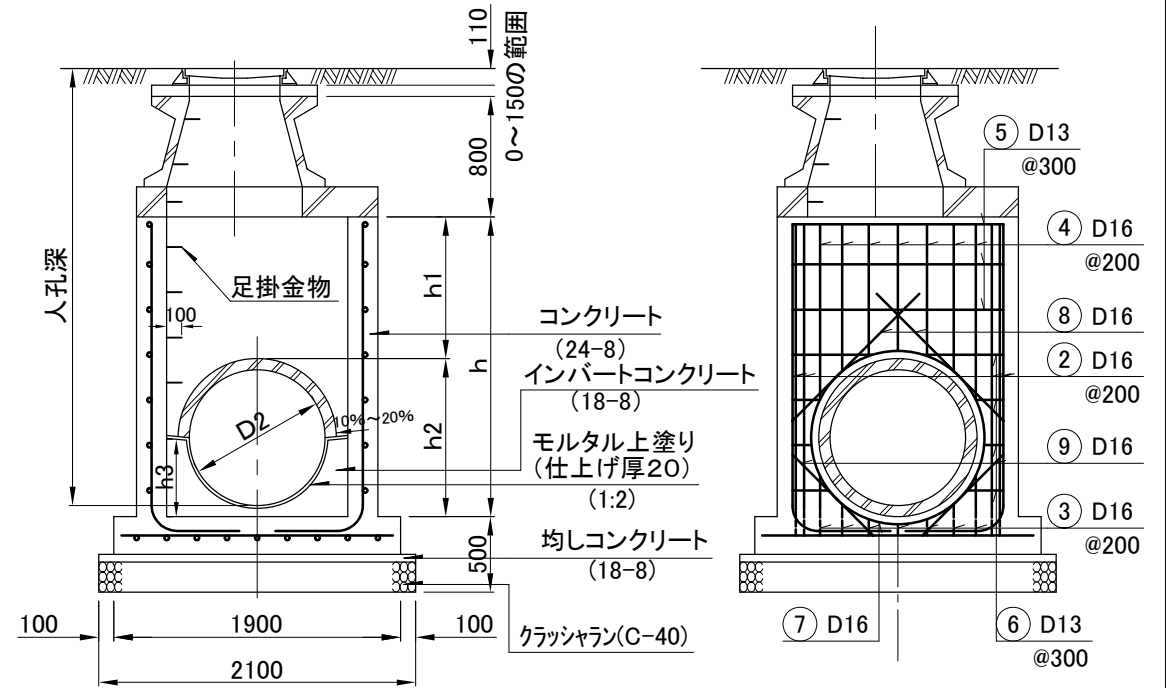
横断面図
