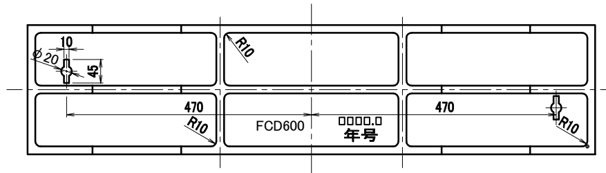
A-A断面図
