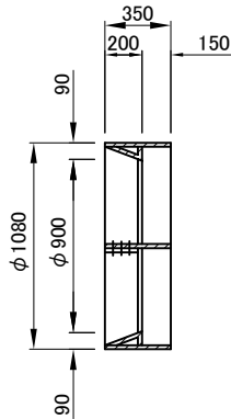
呼び径900mm
