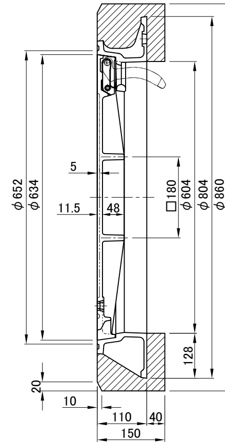
A-A断面図
