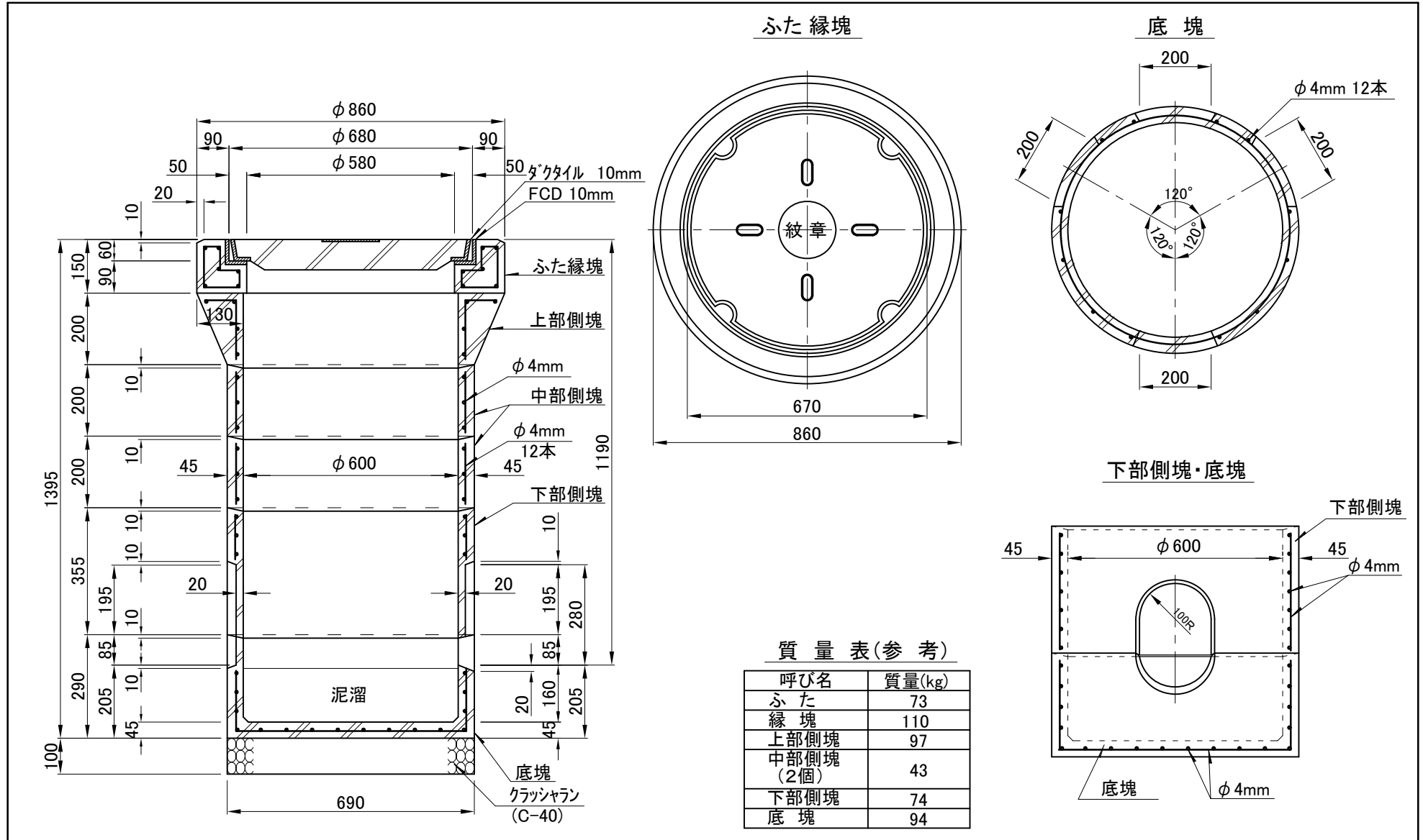
タイプ8接続雨水枺構造図 (φ600)
