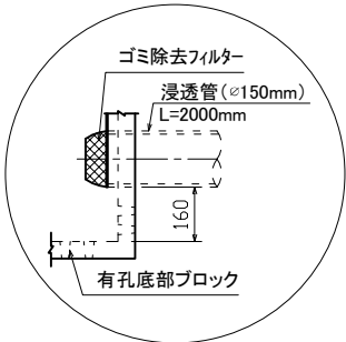
A-A 断面図
