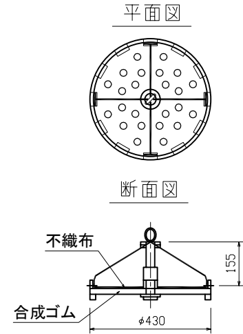
底フィルター図 (参考)
