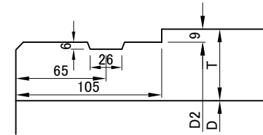
先頭管の管端部詳細
