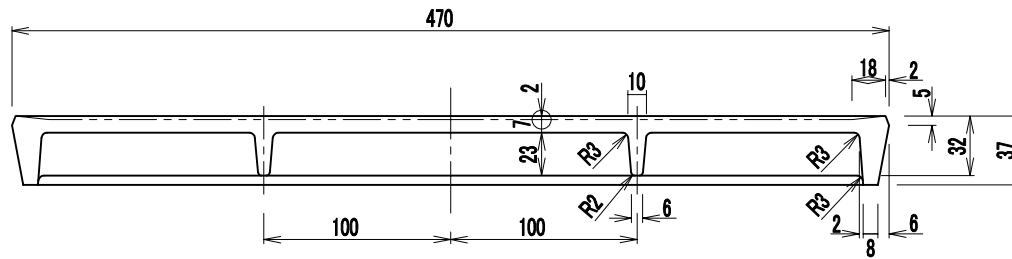
A-A断面図
