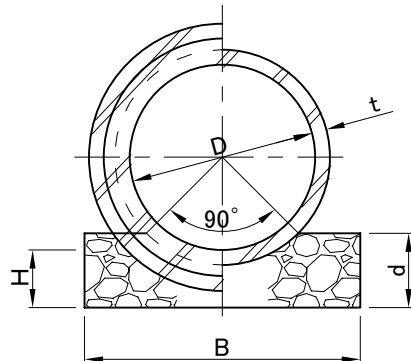
碎石 90° 基礎
