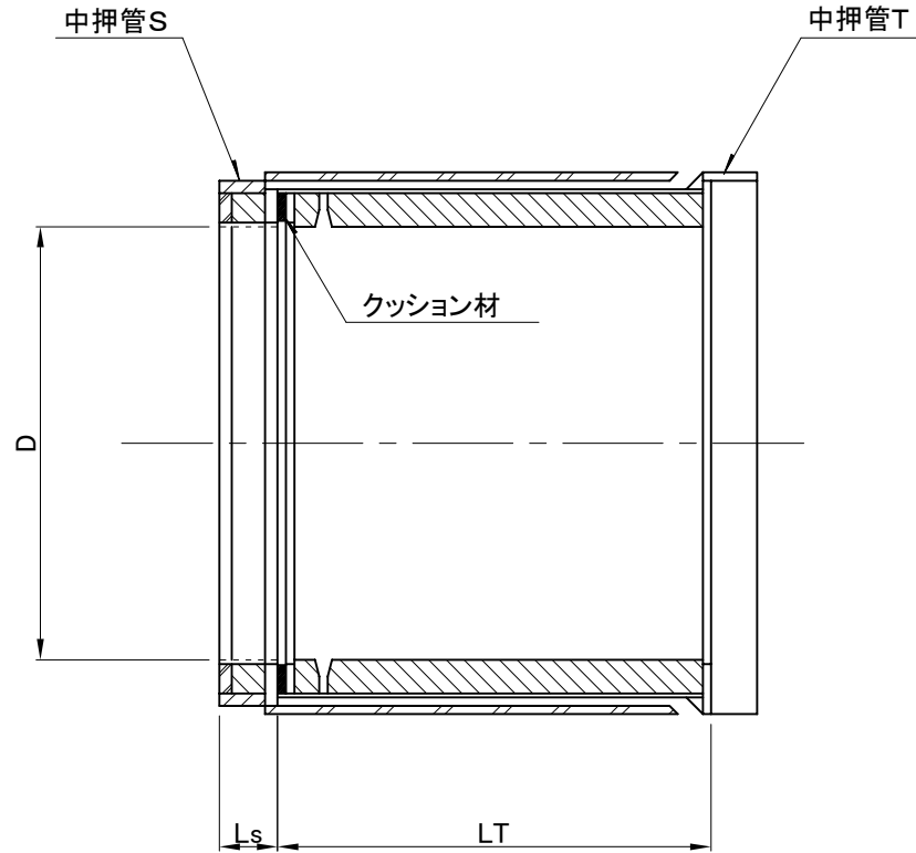
詳細図
