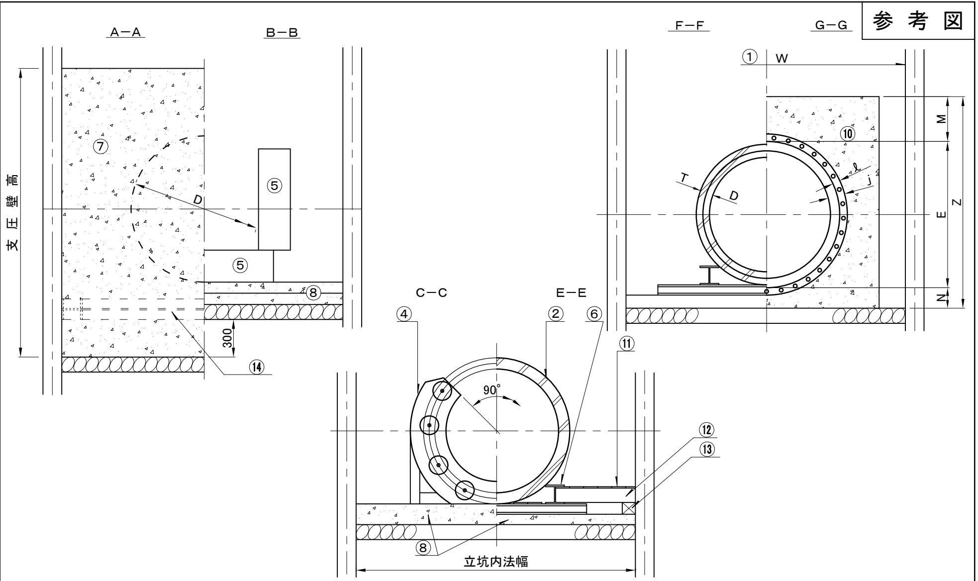
推進設備図(2)
