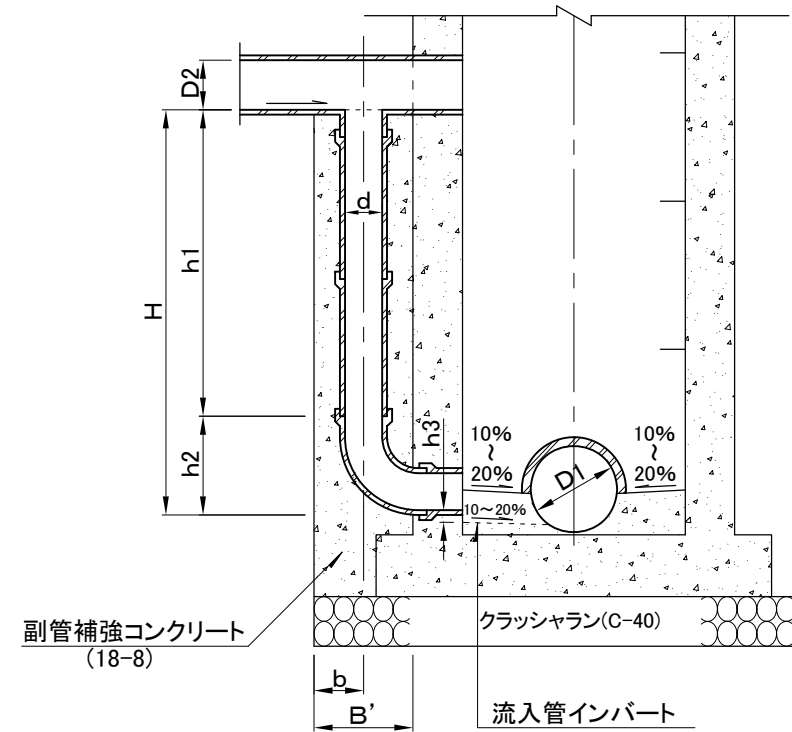
断面図(2)
