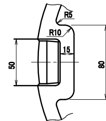
蓋表ボール穴部詳細
