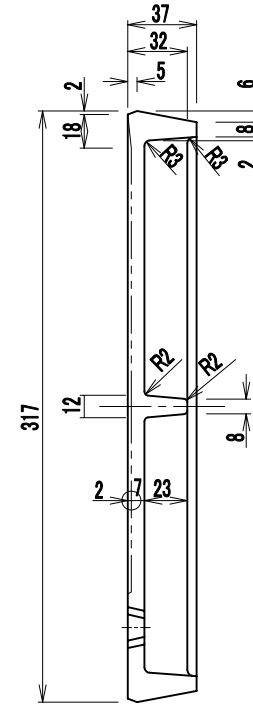
B-B断面図
