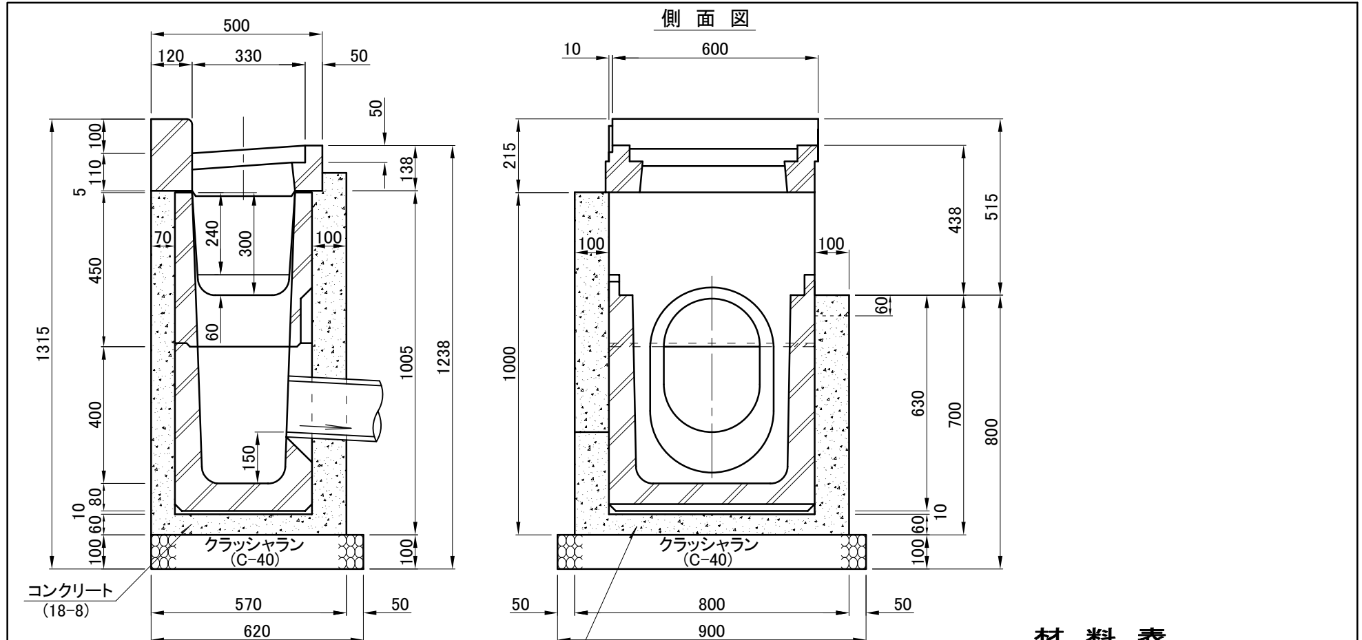
材 料 表
