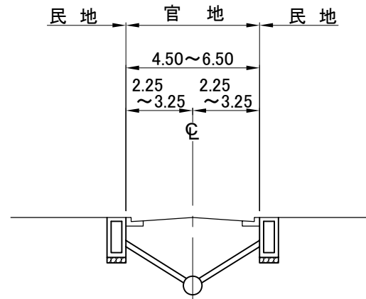
A-A 断面
