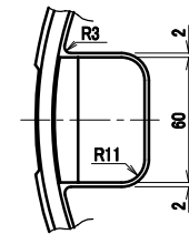
蓋裏ボール穴部詳細
