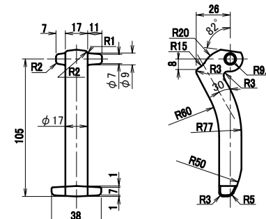
蝶番金物詳細
