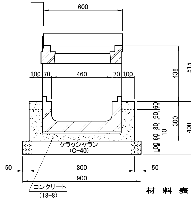
側面図
