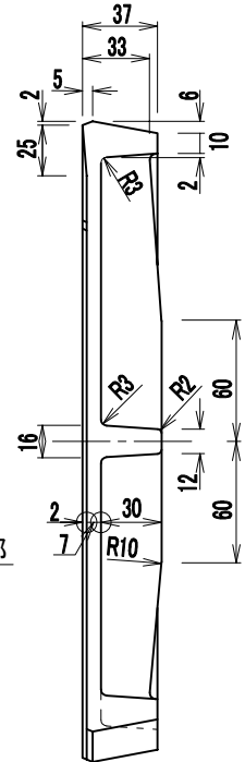
B-B断面図
