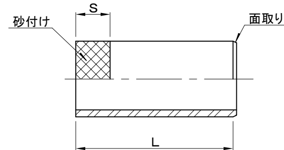
ます取付け継手
