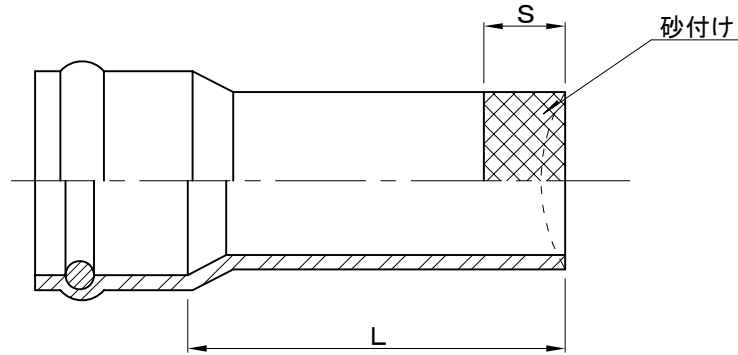
副管分岐用マンホール継手
