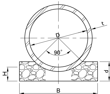
砕石 90° 基礎
