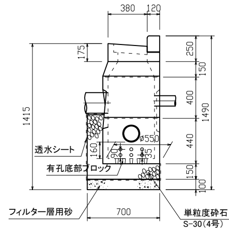
C-C 断面図
