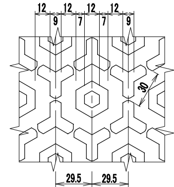
模様詳細図
