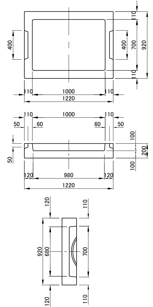
Fブロック構造図
