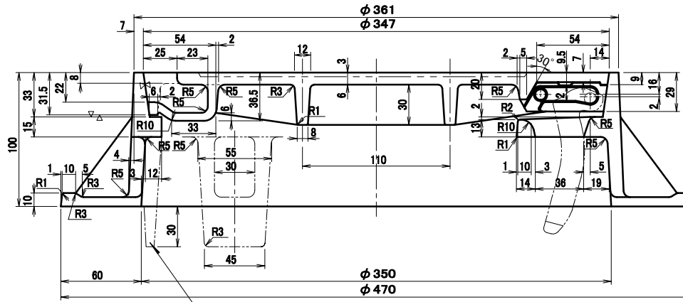
断面
