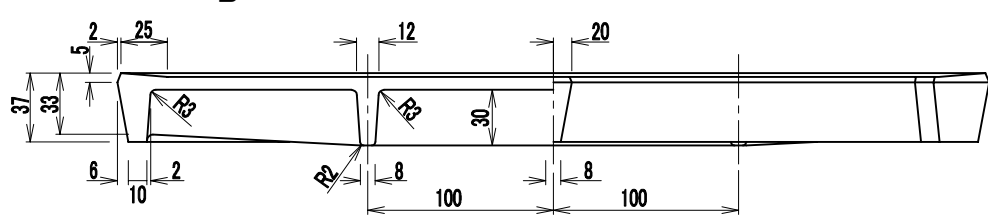
A-A断面図
