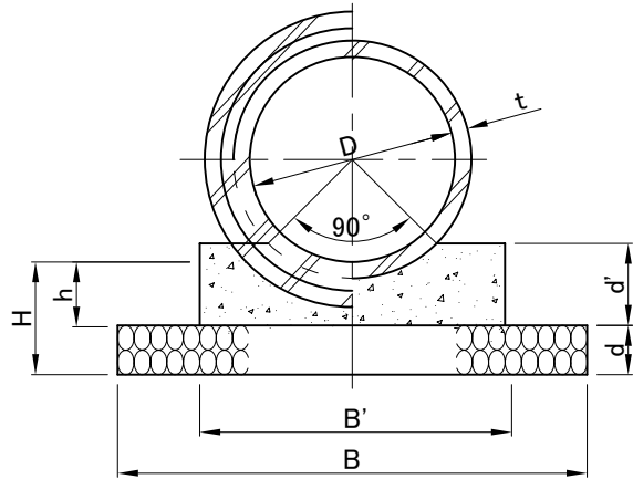
コンクリート 90° 基礎
