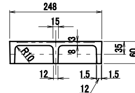
B-B断面図
