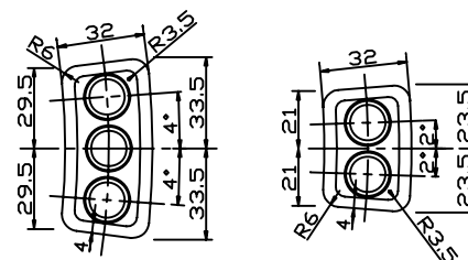
管理番号キャップ取付部詳細
