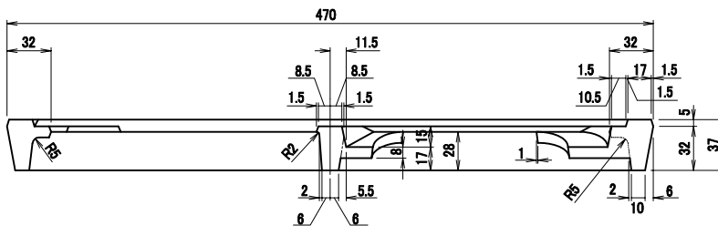
A-A断面図
