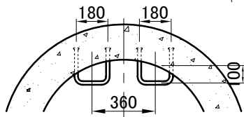
足掛金物詳細図 (ダクティル型)
