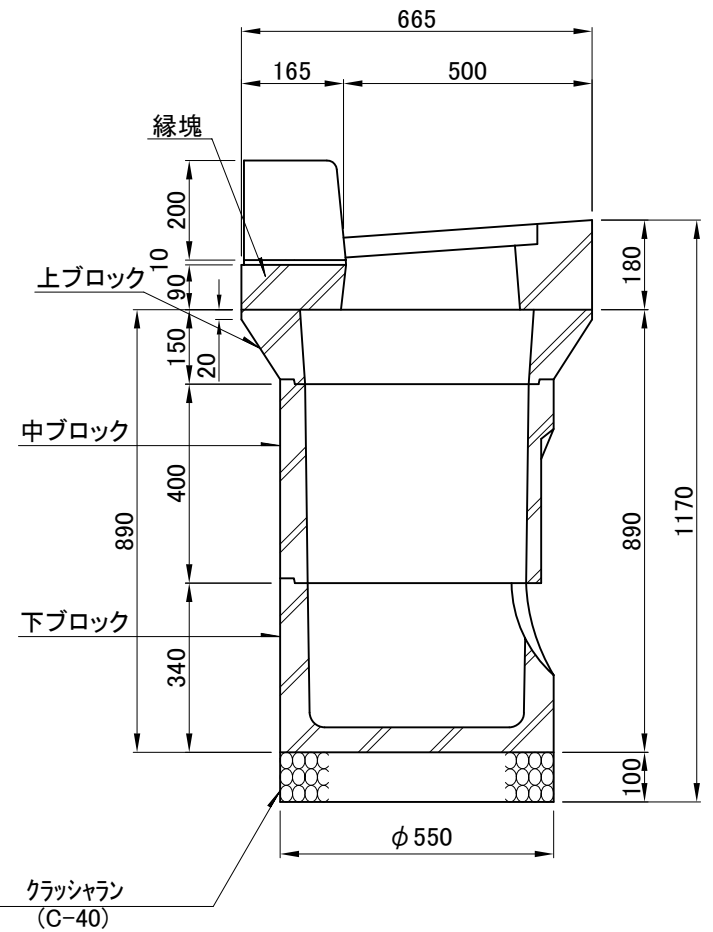
A-A断面図
