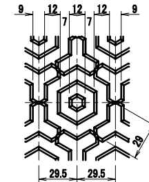
模様詳細
