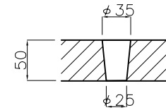
有孔底部ブロック孔詳細図
