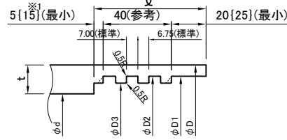
継手受口部詳細図 (Coupling Outlet Detail)
