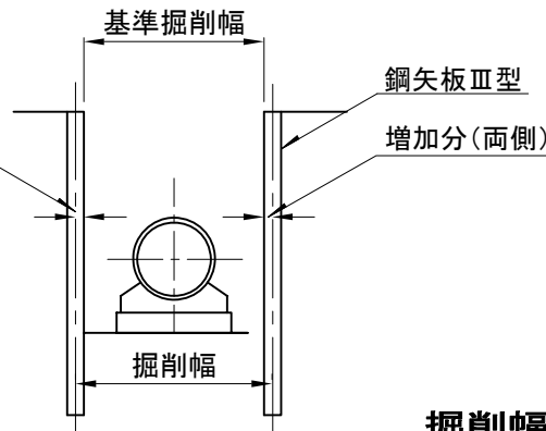
(4) 鋼矢板 III 型
