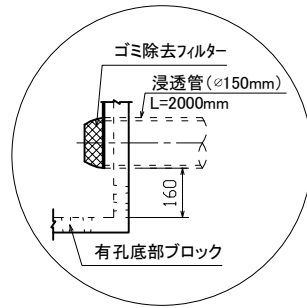
A-A 断面図
