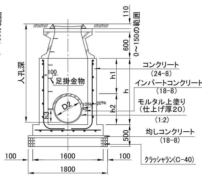
横断面図
