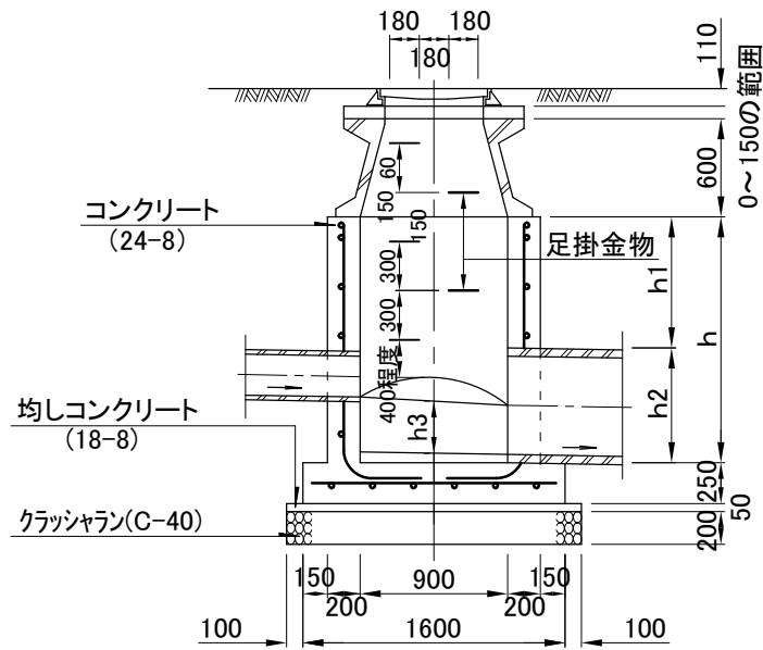
縦断面図
