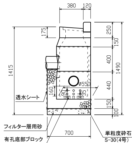
C-C 断面図
