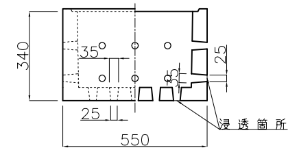
下部側塊
