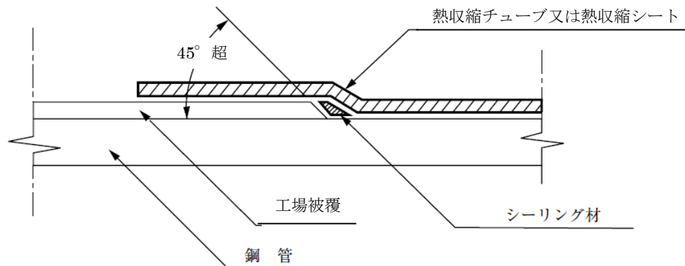
図 2-6 シーリング材の施工
