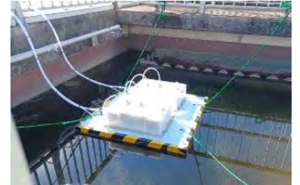
最終沈殿池での N 2 O ガス捕集の様子
