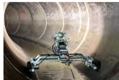
中大口径管用TVカメラの例
