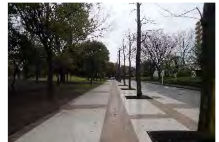
雨水の貯留・浸透機能を有する舗装の整備(中区本牧いずみ公園)
