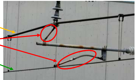
架空電車線と曲線引金物
