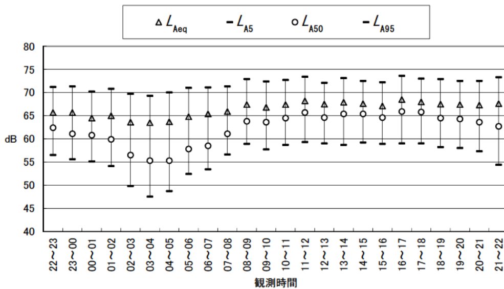
図 3.2-2(4) 道路交通騒音現地調査結果（地点 B：休日）
