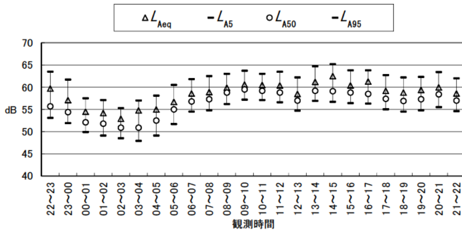
図 3.2-1(1) 環境騒音現地調査結果（地点 b：平日）
