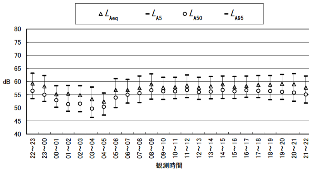
図 3.2-1(2) 環境騒音現地調査結果 (地点 b : 休日)
