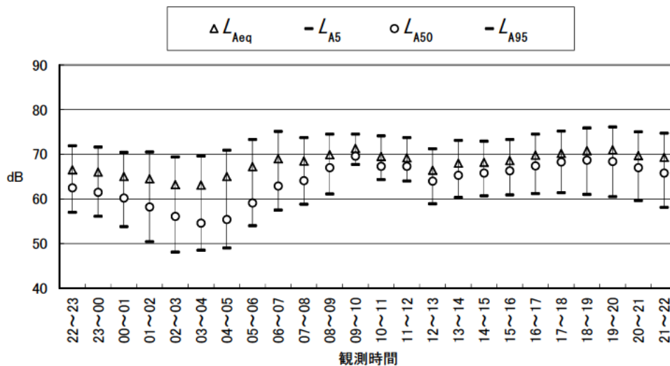
図 3.2-2(3) 道路交通騒音現地調査結果 (地点 B : 平日)
