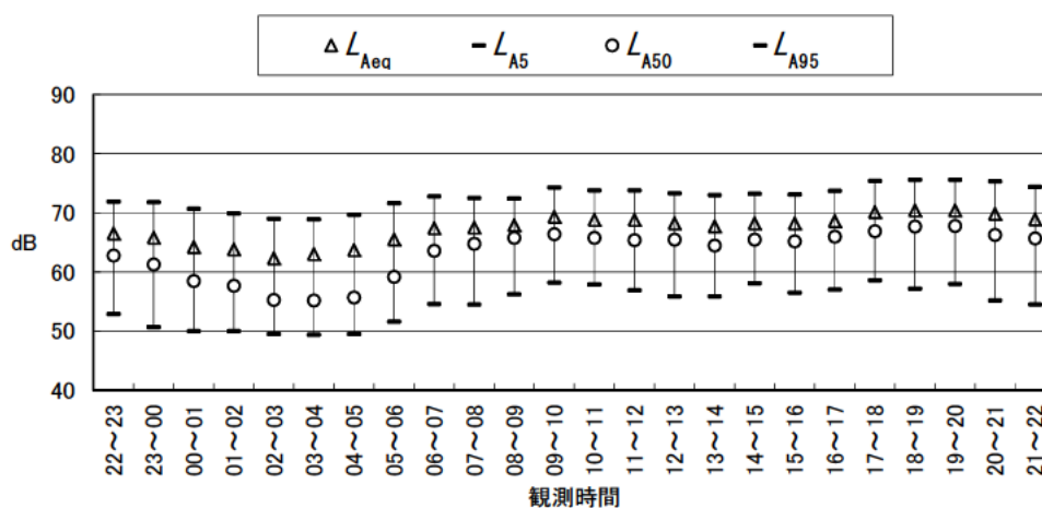
図 3.2-2(1) 道路交通騒音現地調査結果（地点 A：平日）
