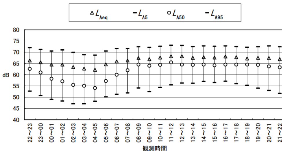
図 3.2-2(2) 道路交通騒音現地調査結果 (地点 A : 休日)
