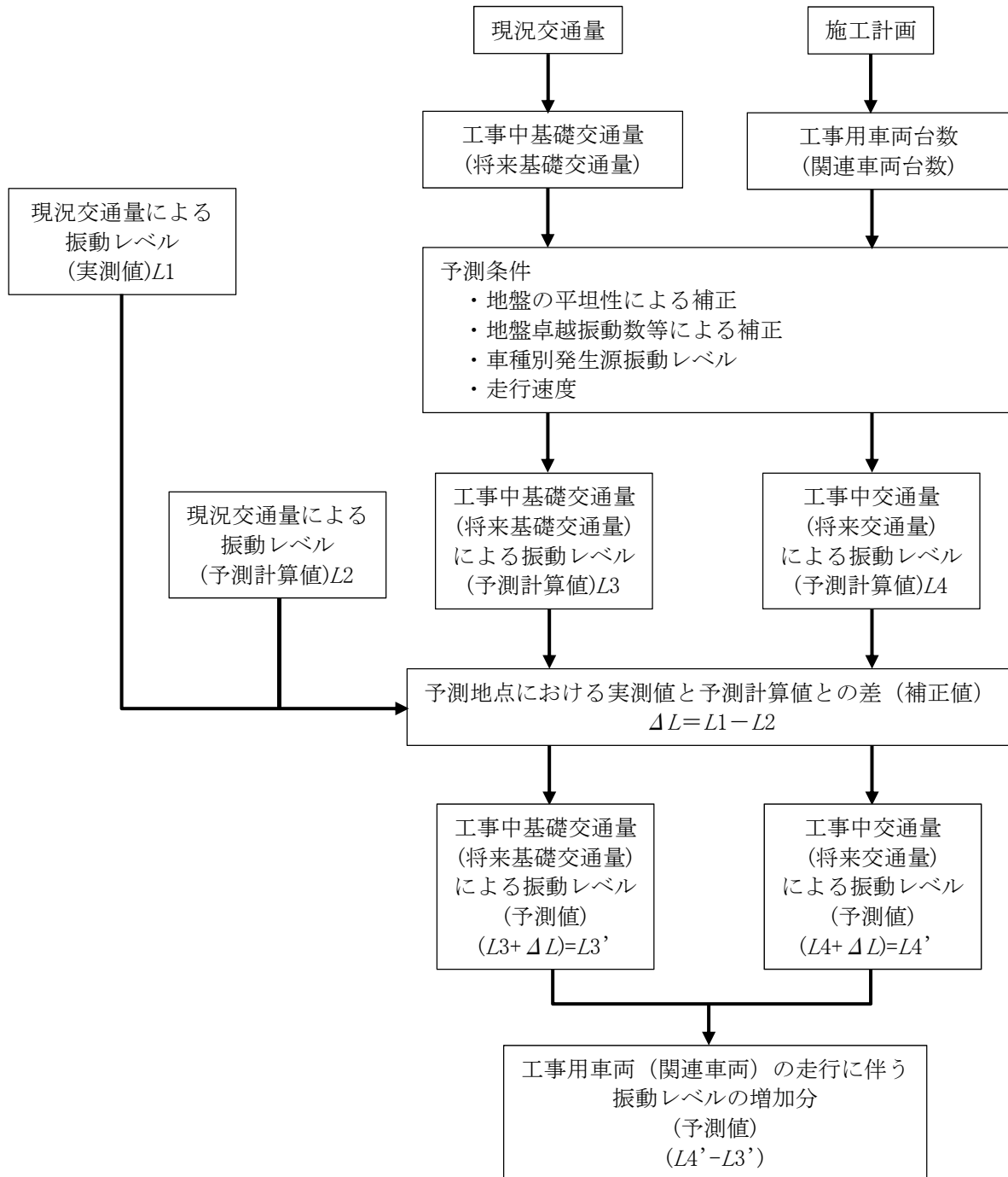
図 6.7-4 予測手順 (工事用車両・関連車両の走行に伴う振動)
