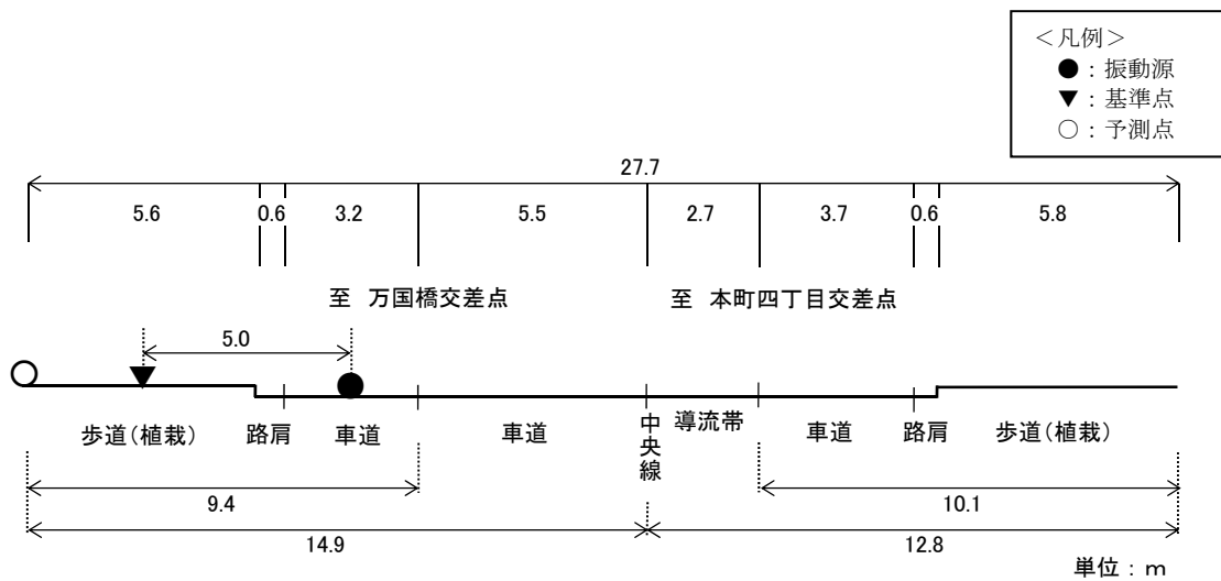
図 6.7-5(1) 道路断面 (地点 A 市道新港 7 号線)
