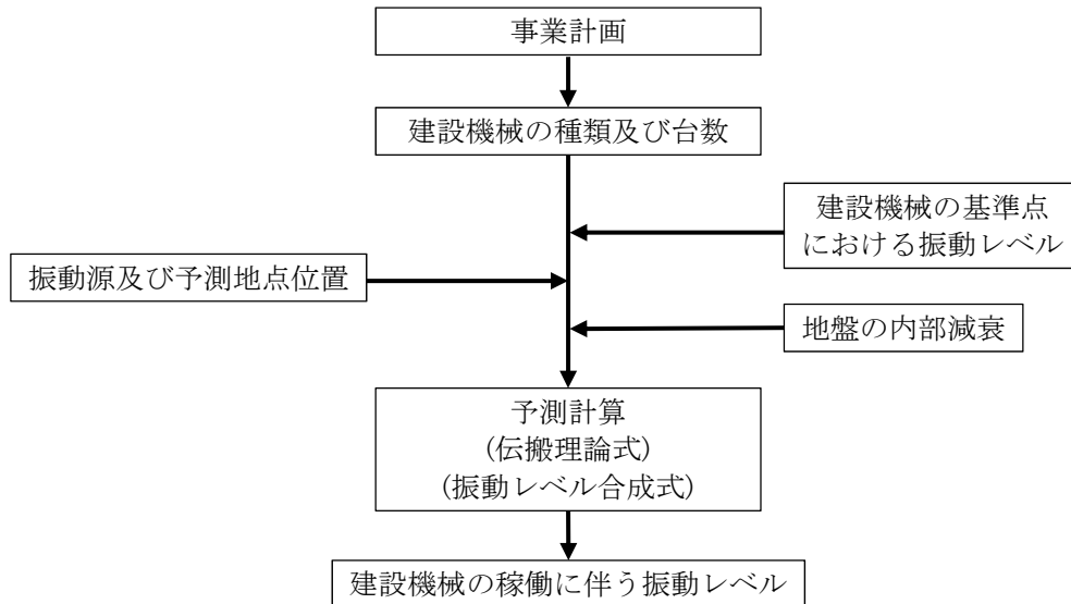
図 6.7-1 予測手順（建設機械の稼働に伴う振動）
