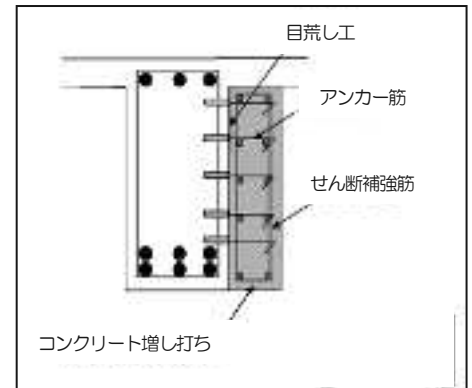
防災対策の例（コンクリート増し打ち）
