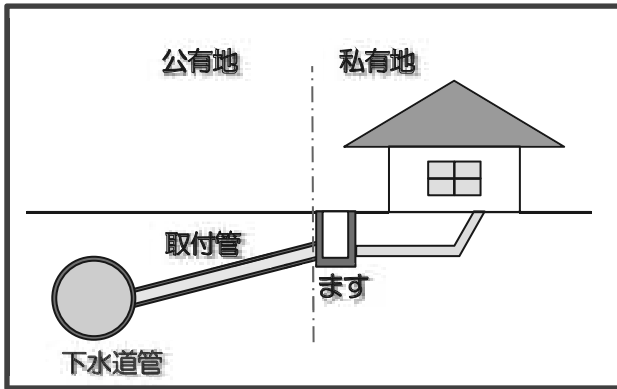
ますと取付管
