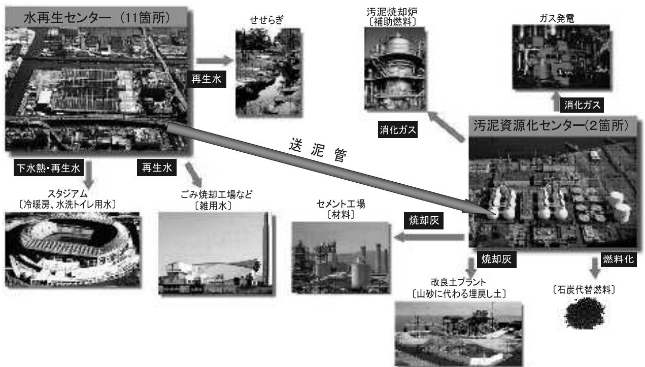
下水道の資源・エネルギー有効利用の流れ
