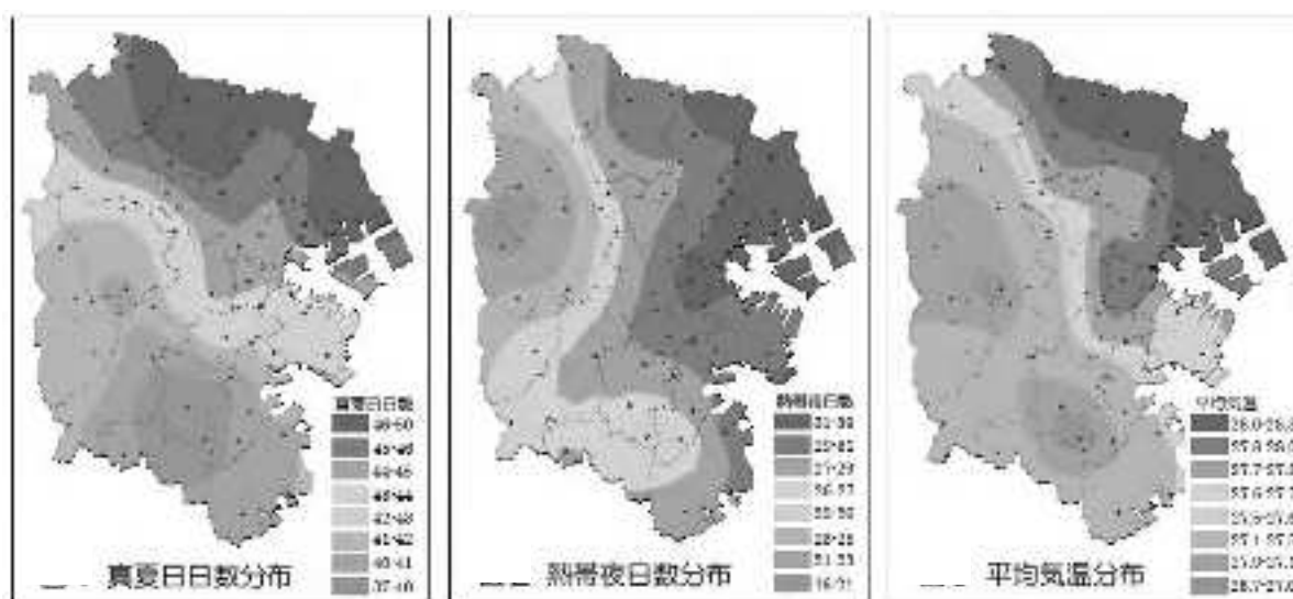
図 平成25年度の観測結果（7～8月、62日 [1,488時間]）
