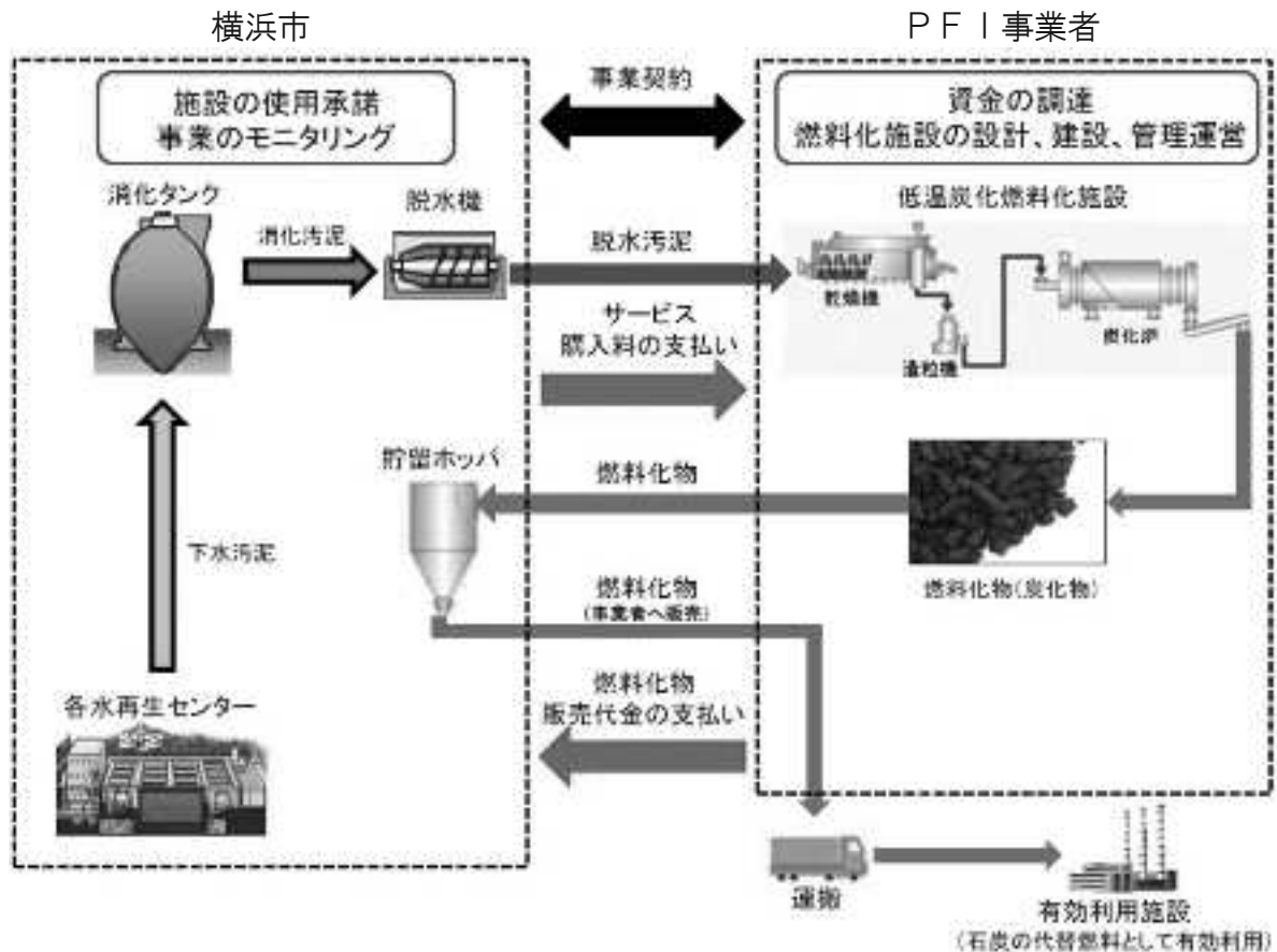
汚泥燃料化事業スキーム
