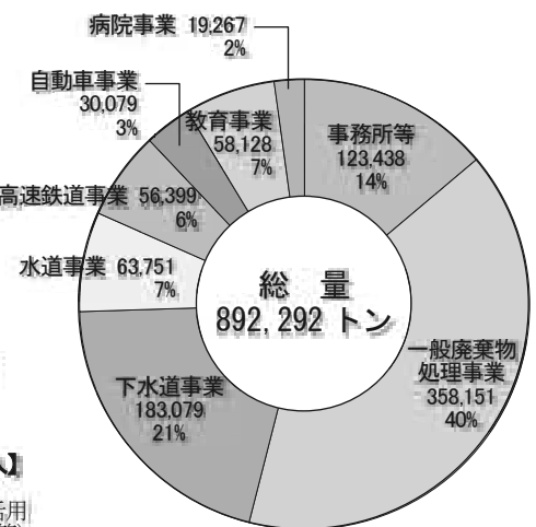
横浜市役所全体(市の事務事業) (平成24年度、単位:t-CO 2 )
