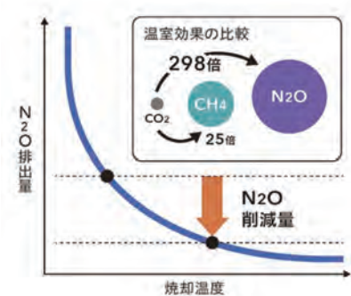
焼却温度とN 2 O排出量の関係
