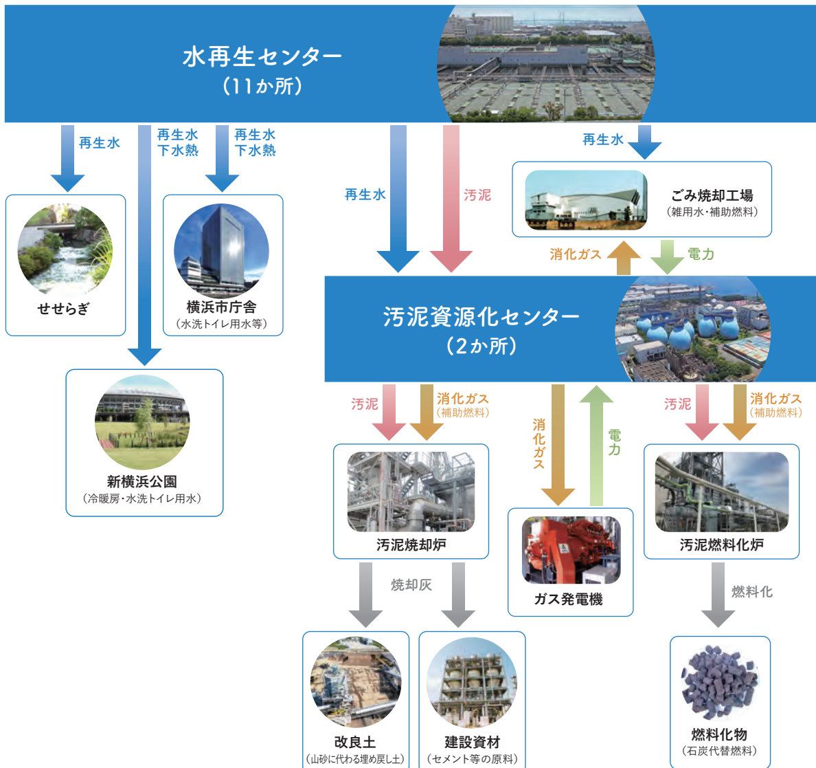
下水道資源の活用フロー
