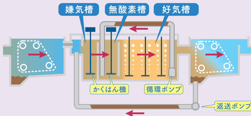
高度処理方式のイメージ A2O法(嫌気・無酸素・好気法)
