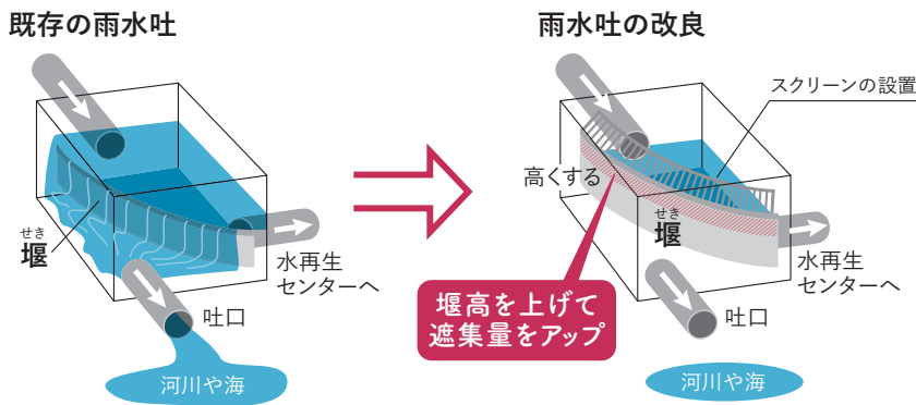
雨水吐の改良イメージ
