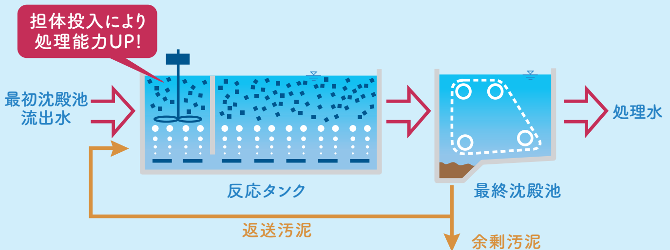
下水処理能力増強技術<担体投入型活性汚泥法>
